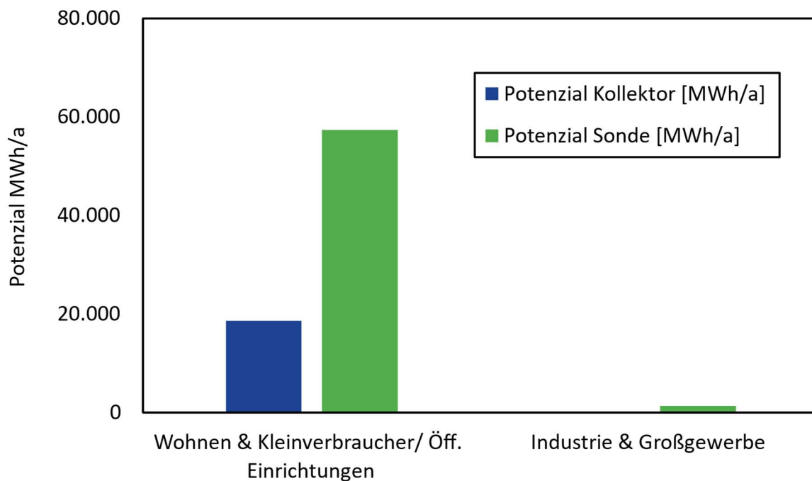
Abbildung 4: Potenzial Wärme aus oberflächennaher Geothermie
