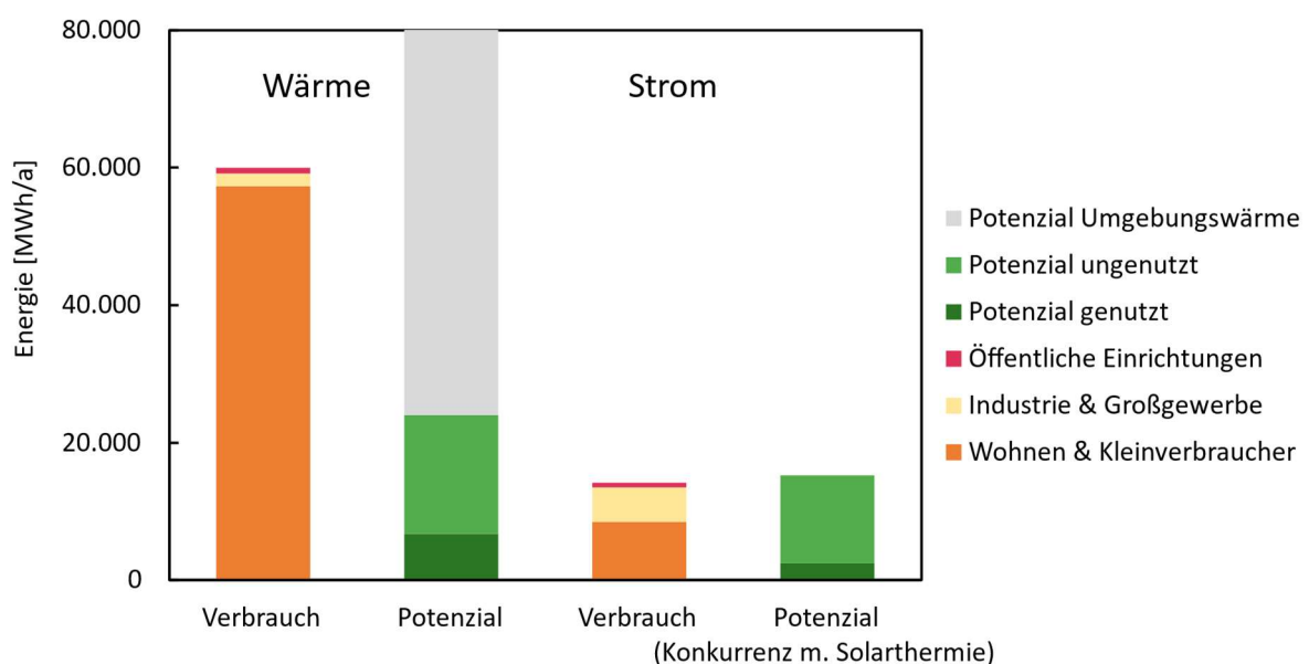
Abbildung 13: Gegenüberstellung Verbrauch und Potenzial von Wärme und Strom
