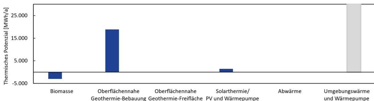
Abbildung 9: Zusammenfassung Potenziale erneuerbarer Wärme
