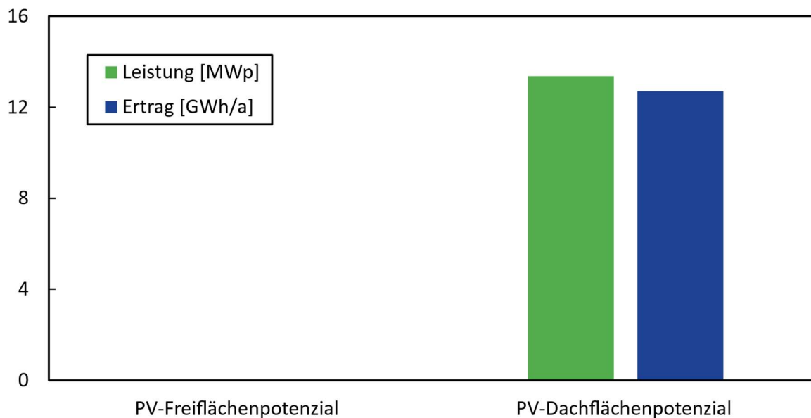
Abbildung 10: Potenzial Leistung und Ertrag Photovoltaik
